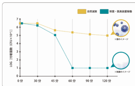
空間除菌性能の試験結果
