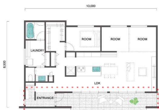
玄関からリビングが見えないように配置したプラン例 ※図面下部赤枠部分がミッドテリア
