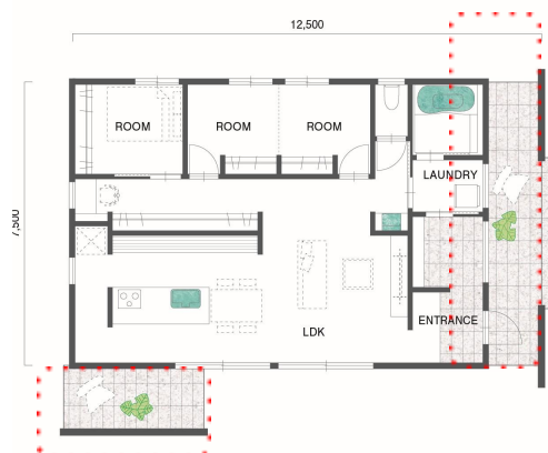
土間収納を大きく取り、2か所にミッドテリアを設けたプラン例 ※図面右側と下側の赤枠部分がミッドテリア
